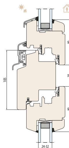
SISTEMA NATURO 68 Traverso 105 mm
