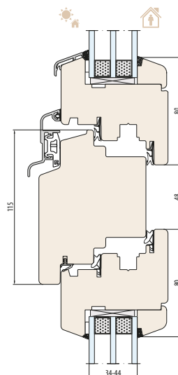
SISTEMA NATURO 80 Traverso 115 mm
