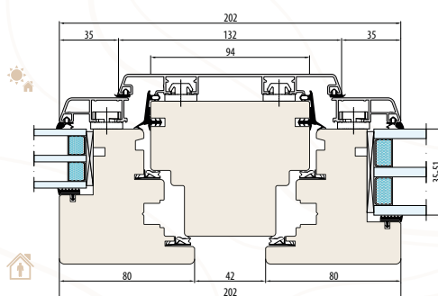
Montante fisso 94 mm (Sezione orizzontale)
