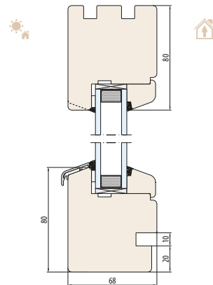
SISTEMA NATURO 68-FIX Scanalatura per davanzale interno
