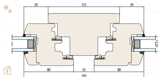
SISTEMA NATURO 68 Montante fisso 115 mm (Sezione orizzontale)
