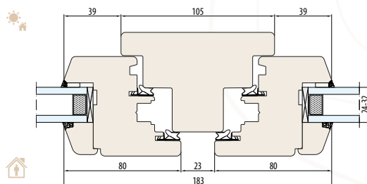
SISTEMA NATURO 68 Montante fisso 105 mm (Sezione orizzontale)
